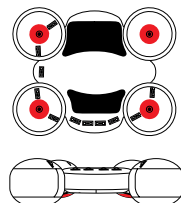
ION
